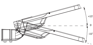
Instalación Horizontal ±0-5-10-15°
